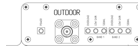
Панель индикации
