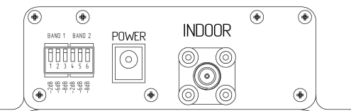
Панель настройки
