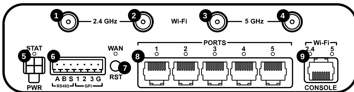
Рис. 2. Вид спереди
